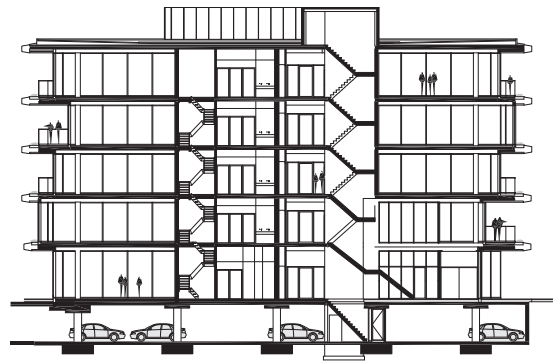
doorsnede
