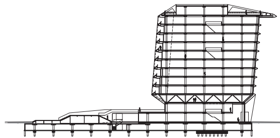
langsdoorsnede
