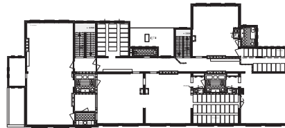
eerste verdieping
