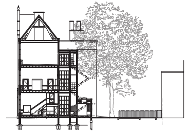
doorsnede
