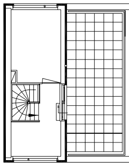
type A, 2e verdieping
