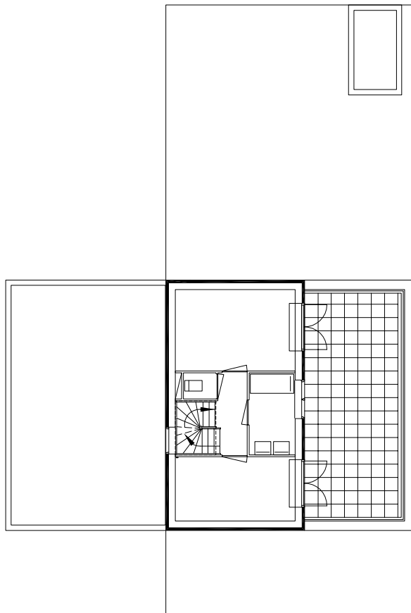
type D, 1e verdieping
