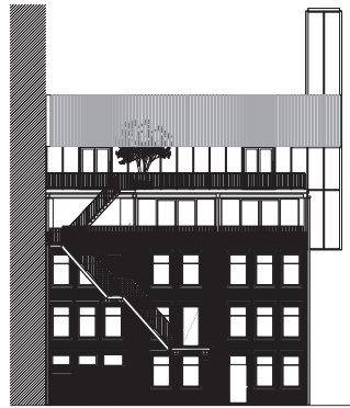
achtergevel
