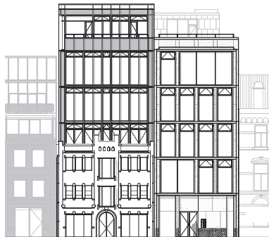
noordgevel
