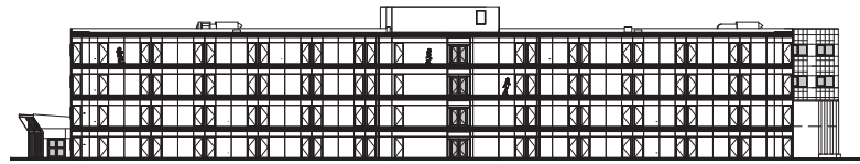
doorsnede
