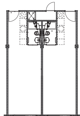
verdieping
