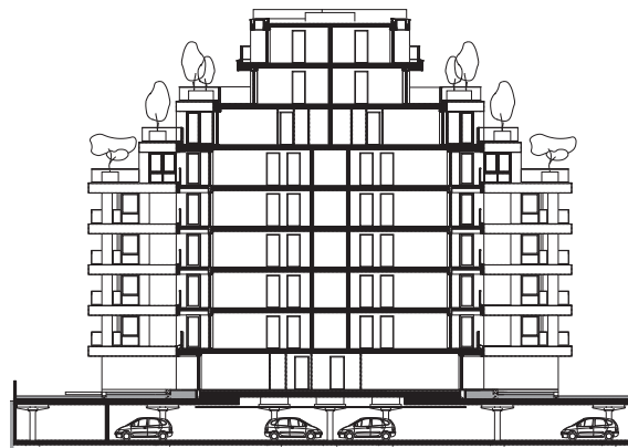
doorsnede
