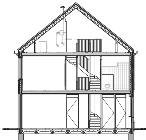
doorsnede
