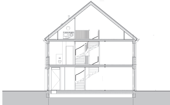
doorsnede
