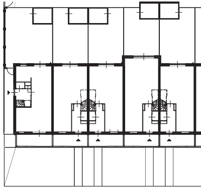
situatie begane grond
