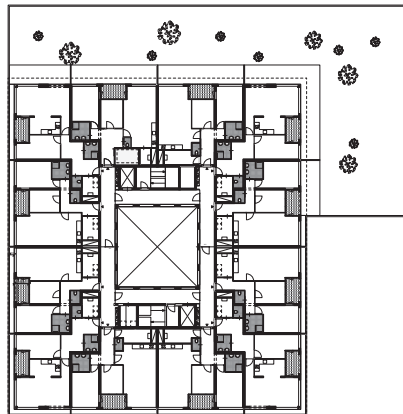
vijfde verdieping
