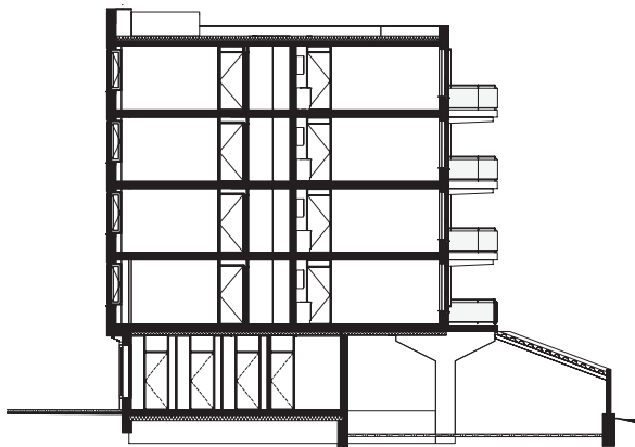
doorsnede
