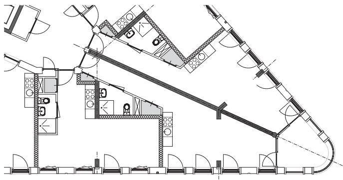
plattegrond hoekwoning
