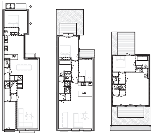
begane grond, eerste en derde verdieping
