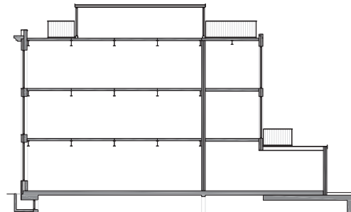
langsdoorsnede
