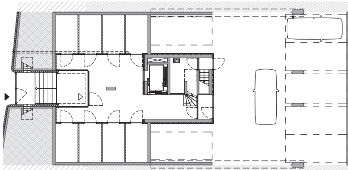
begane grond
