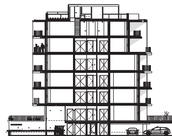
doorsnede
