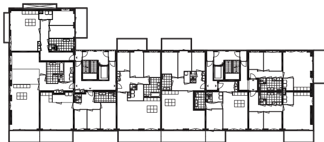
derde verdieping
