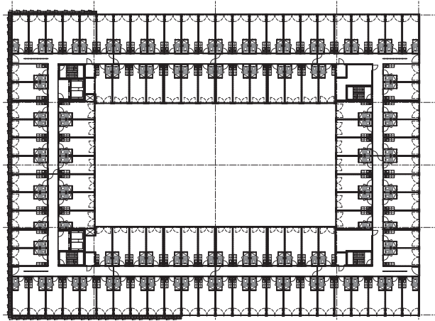
begane grond
