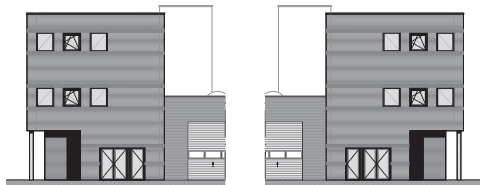
rechter en linker zijgevel
