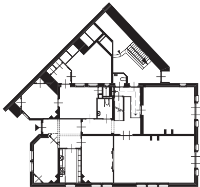
begane grond
