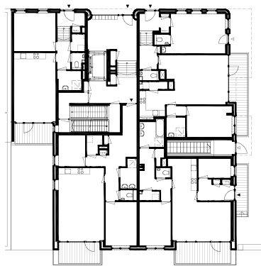
begane grond
