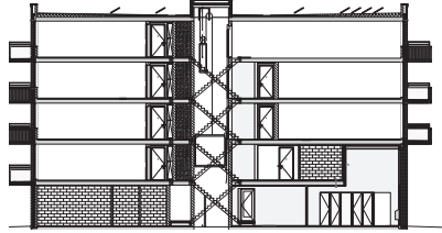
doorsnede
