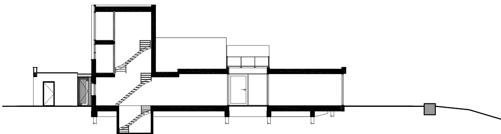
doorsnede type 2
