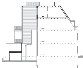
doorsnede
