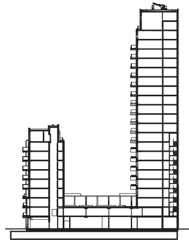
doorsnede
