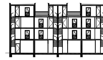
doorsnede C-C
