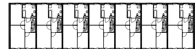
2e verdieping / 6.400+P
