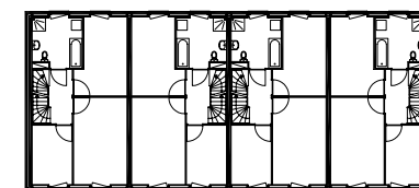
2e verdieping / 6.400+P
