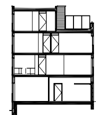
doorsnede B-B
