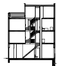
doorsnede A-A
