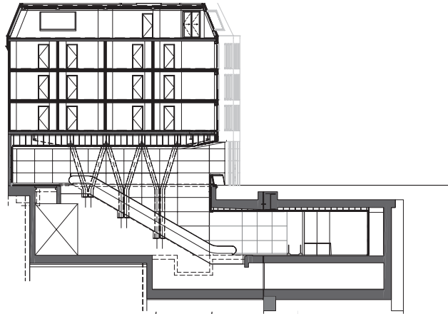
doorsnede
