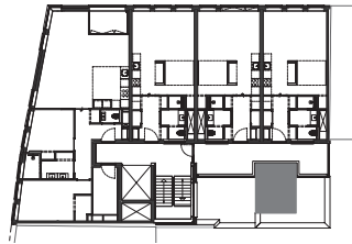
begane grond
