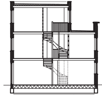
doorsnede
