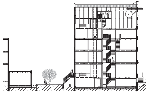
doorsnede Prinsengracht 693
