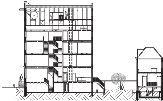
doorsnede Prinsengracht 691
