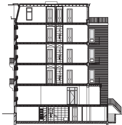
doorsnede
