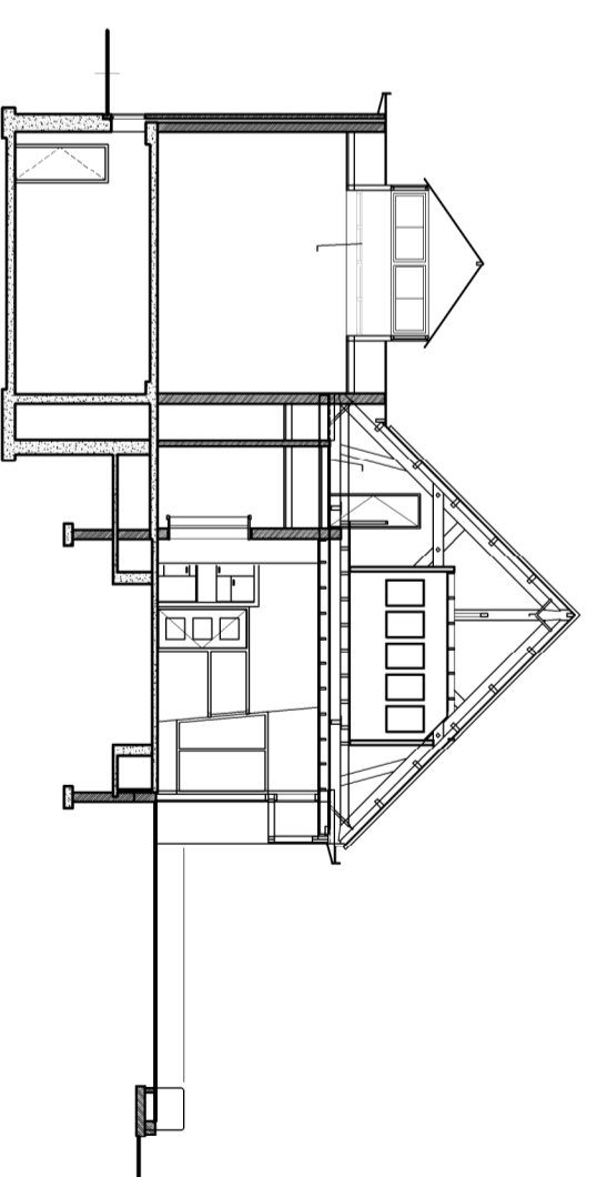
doorsnede C
