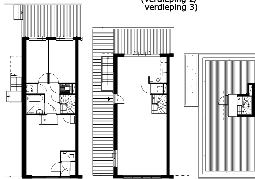
Woning 4 (begane grond/verdieping 1/verdieping 2)
