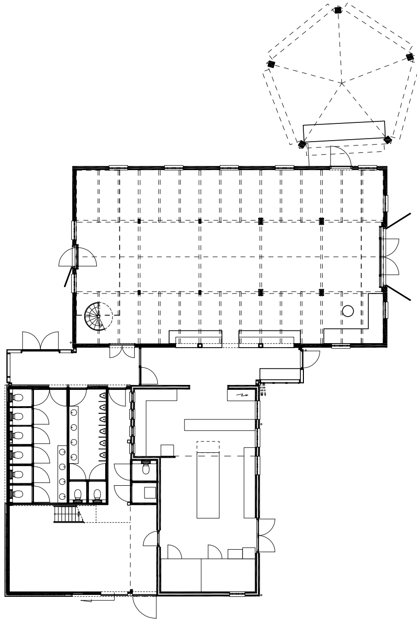
plattegrond
