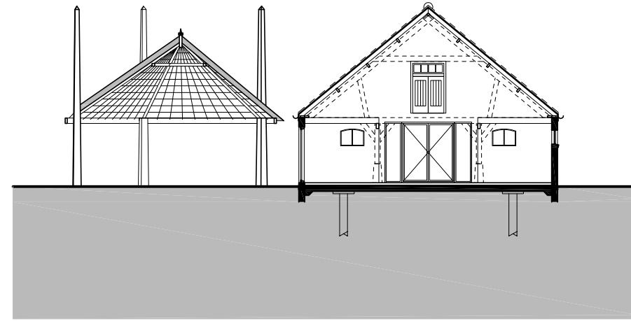
doorsnede restaurant / hooibarg
