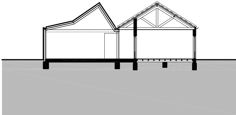
doorsnede keuken / uitbreiding
