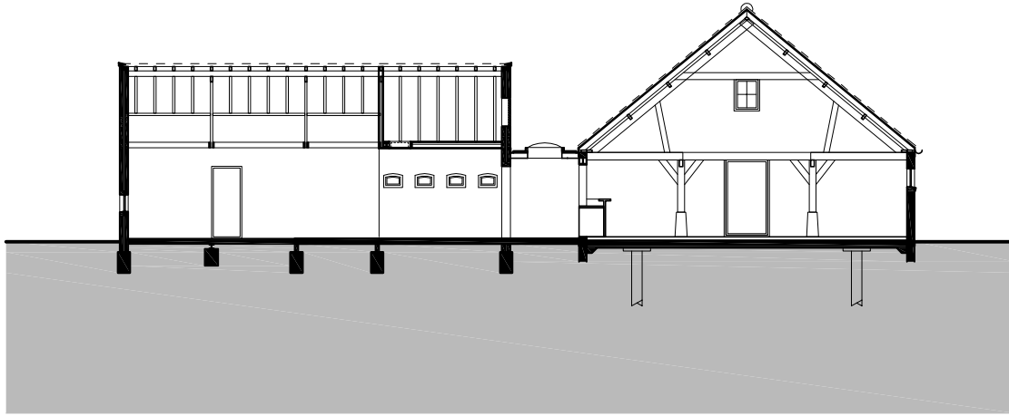
doorsnede restaurant / keuken
