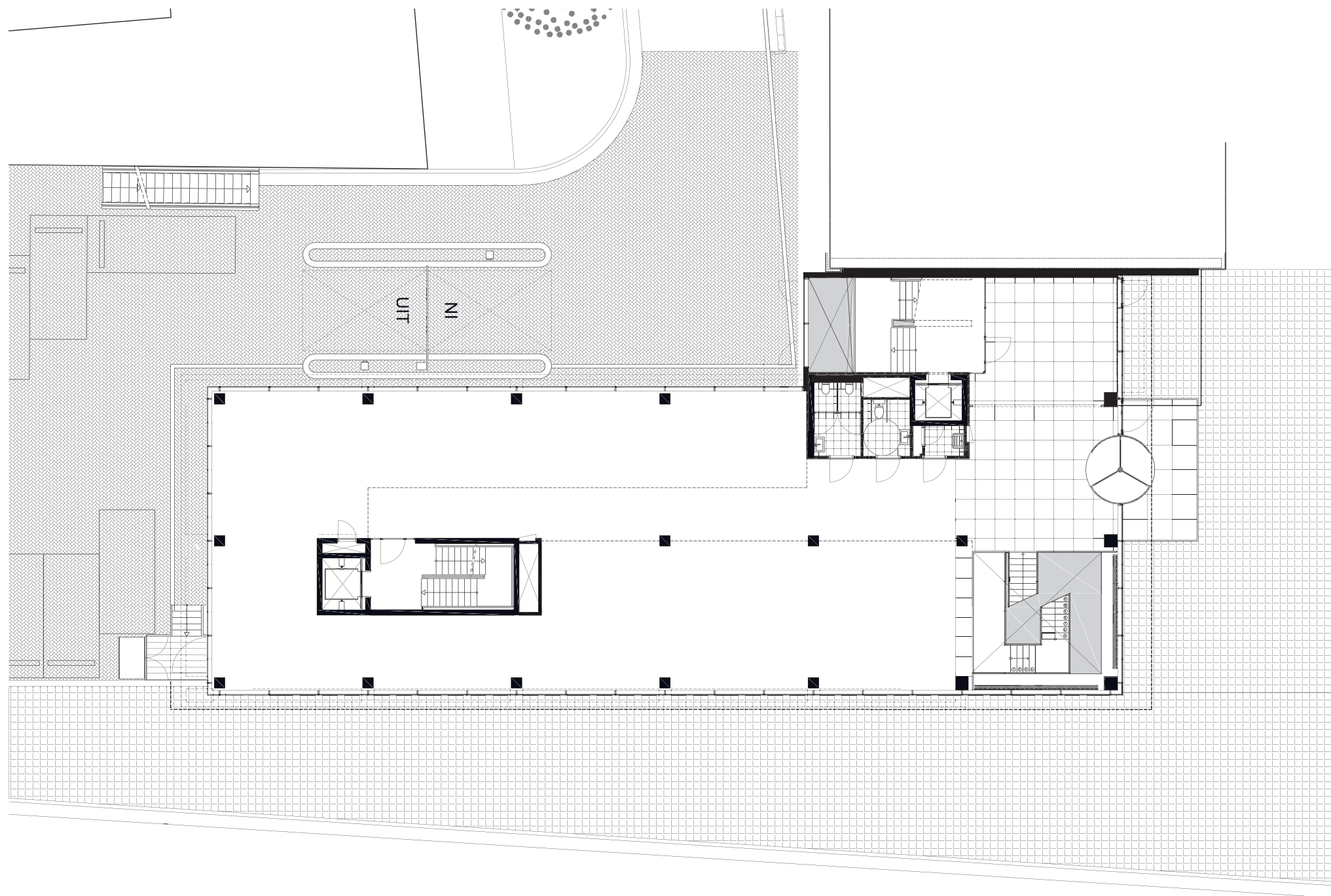
VALINA plattegrond begane grond SCHAAL 1:200
