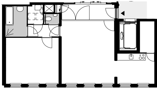
WONINGTYPE H1
