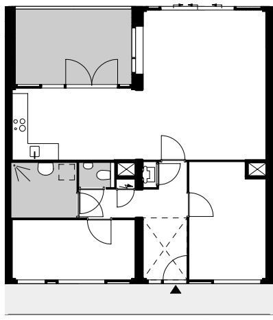
WONINGTYPE P1
