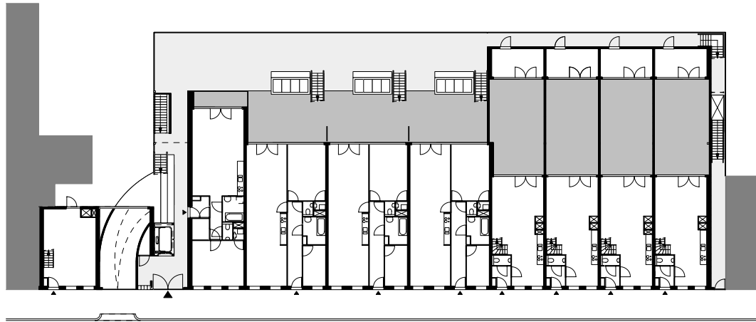
BEGANE GROND
