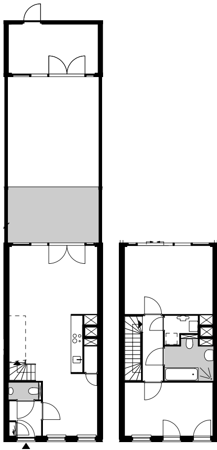
WONINGTYPE E1
