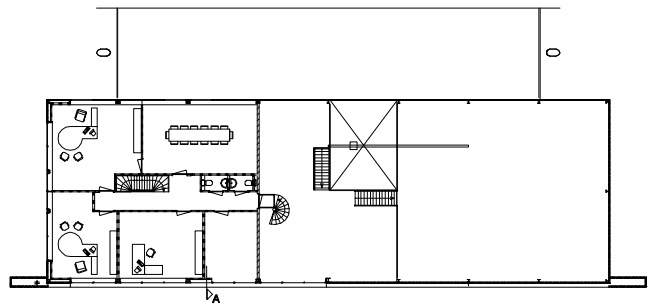
2E VERDIEPING
