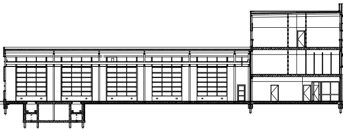
DOORSNEDE A-A
