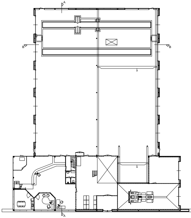
BEGANE GROND
