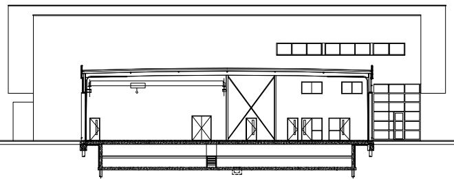
DOORSNEDE B-B
