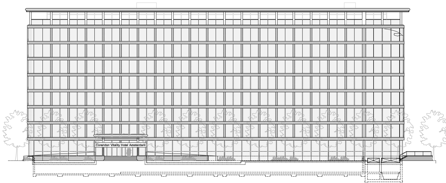
Noordgevel
