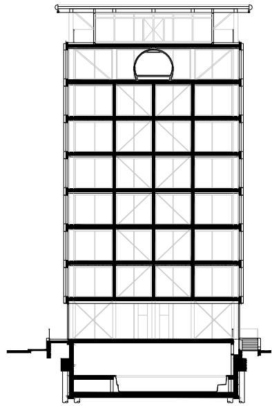
Doorsnede B-B
