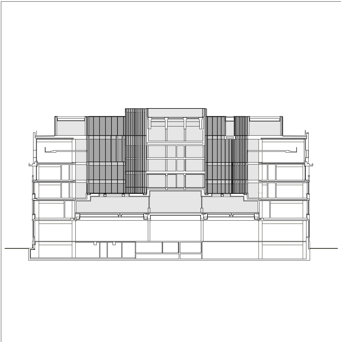
W hotel, 'Exchange' gebouw, Amsterdam doorsnede
