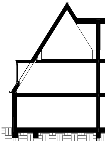
doorsnede type L
