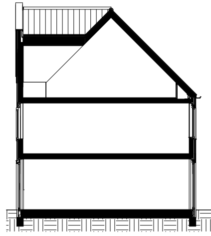
doorsnede type N
