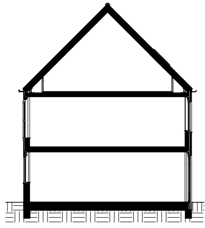
doorsnede type C
