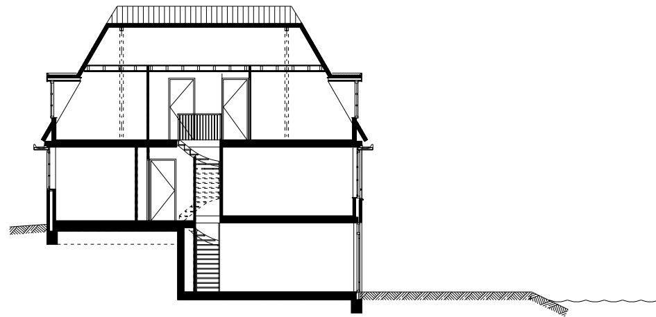
Doorsnede 02
