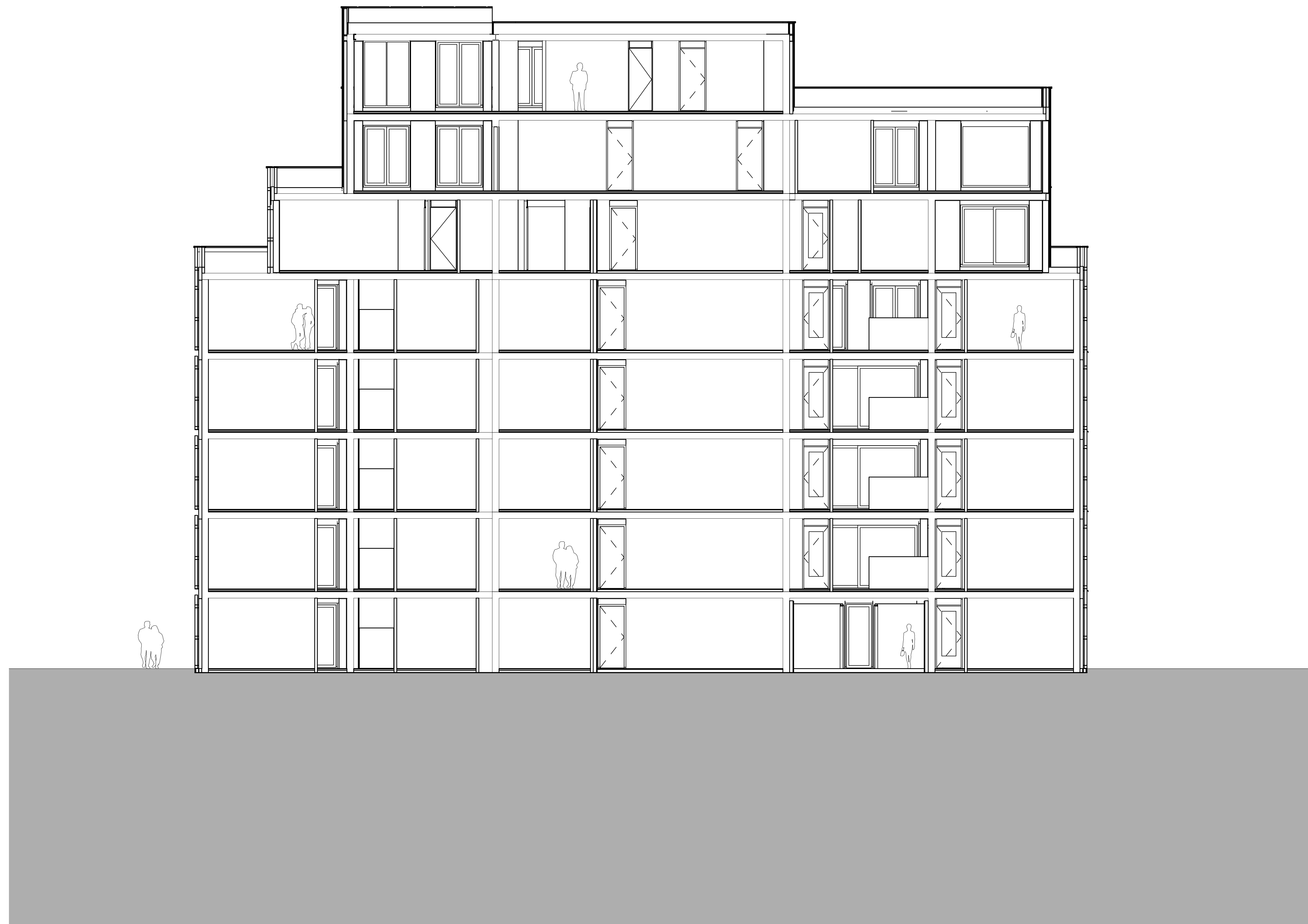
Doorsnede D
