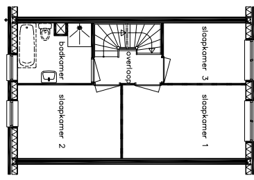
1e verdieping
