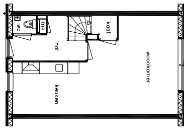
begane grond
