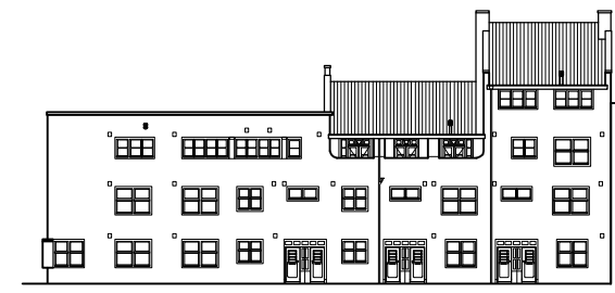
Ringdijk Voorgevel
