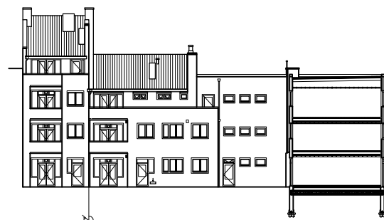
Ringdijk Achtergevel
