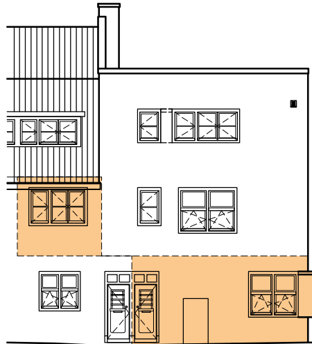
VOORGEVEL
