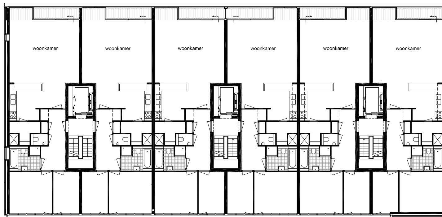
Woningplattegronden Kostverlorenvaart 1e, 2e, 3e verdieping 1: 200
