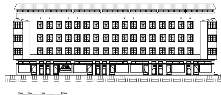
Voorgevel Niasstraat (zuid)
