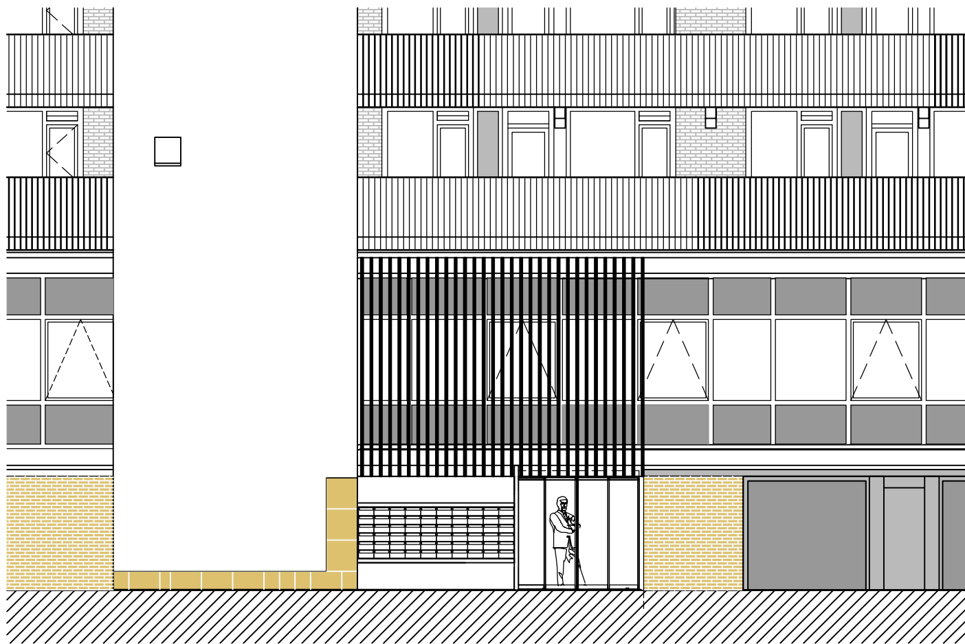
AANZICHT ENTREE WONINGEN
