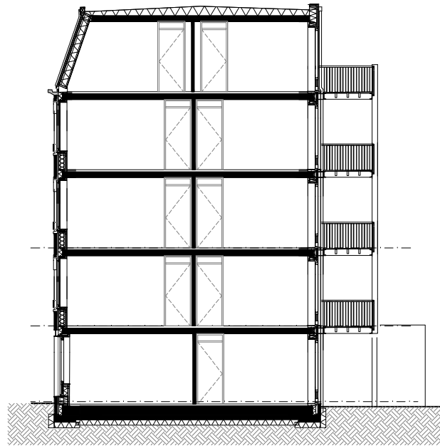
doorsnede
