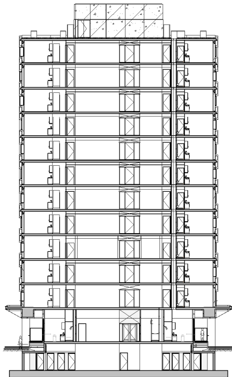
doorsnede A
